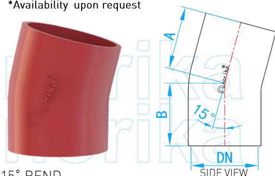
15° BEND
