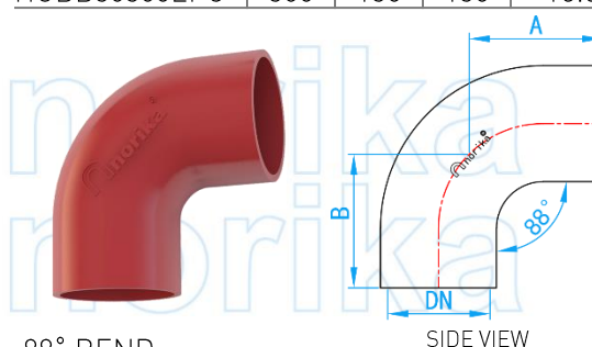
88° BEND
