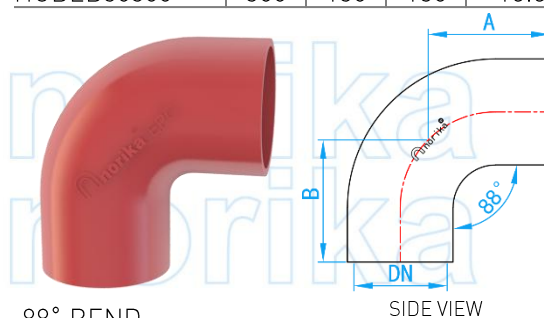
88° BEND
