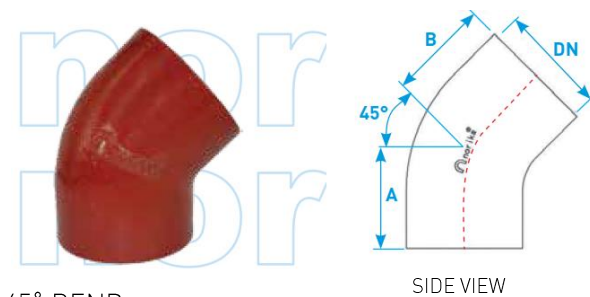
45° BEND
