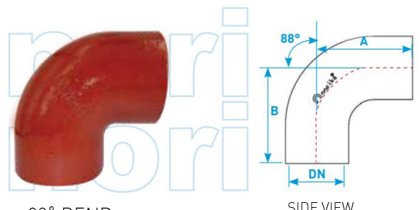
90° BEND
