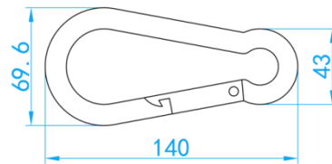
AISI316 Carabiner
